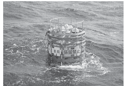
浮魚礁
