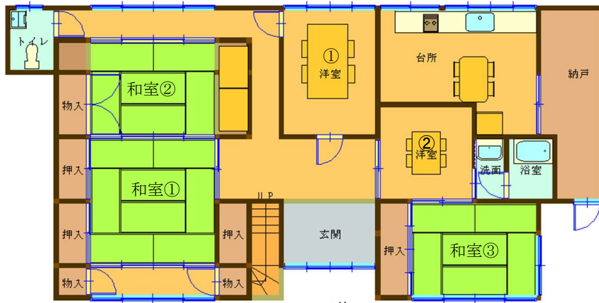
1 階
